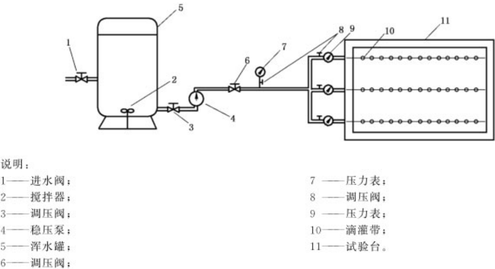
图 2 抗泥沙堵塞性能试验装置示意图
